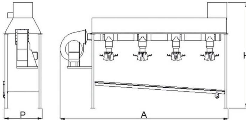
FOCALIZADORA 4 BOCAS
